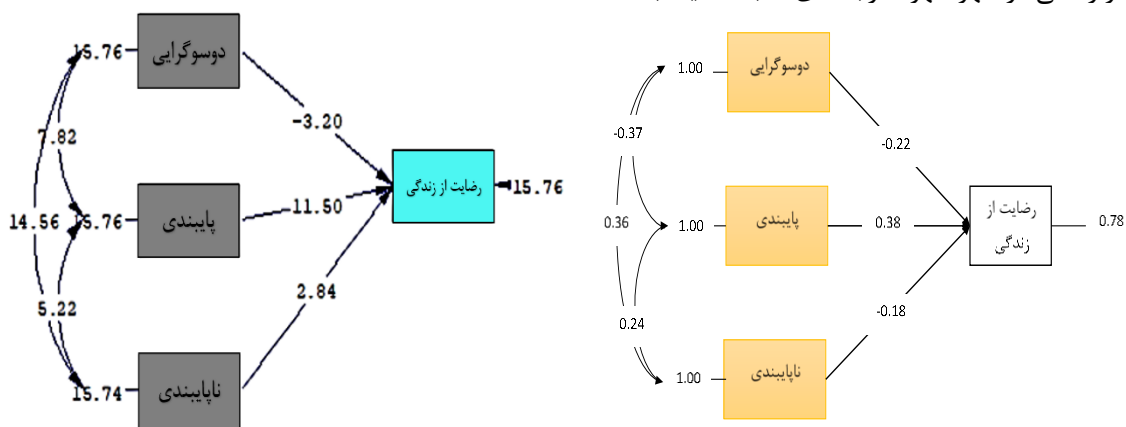
شکل ۱. مدل معادلات ساختاری فرضیه اول بر اساس مقادیر بار استاندارد شده (سمت راست) و مقدار T (سمت چپ)
