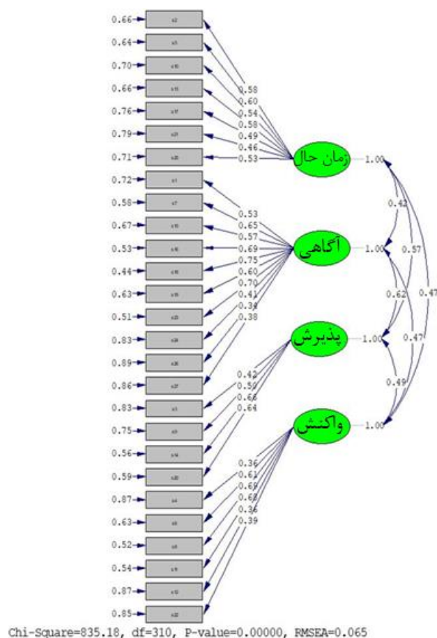
شکل ۱. نمودار تحلیل عاملی تأییدی
